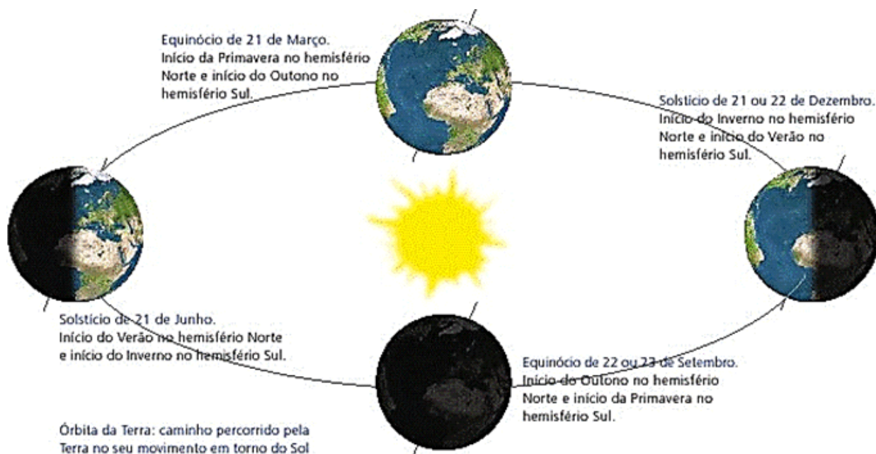
Figura 1: O movimento de translação da Terra e as estações do ano.
